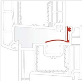
Lüfterstellung bei normalem Luftdruck
