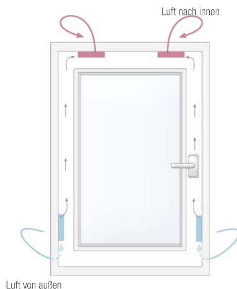
Bei steigendem Winddruck schließt der AirComfort automatisch nach dem Bernoulli-Prinzip
